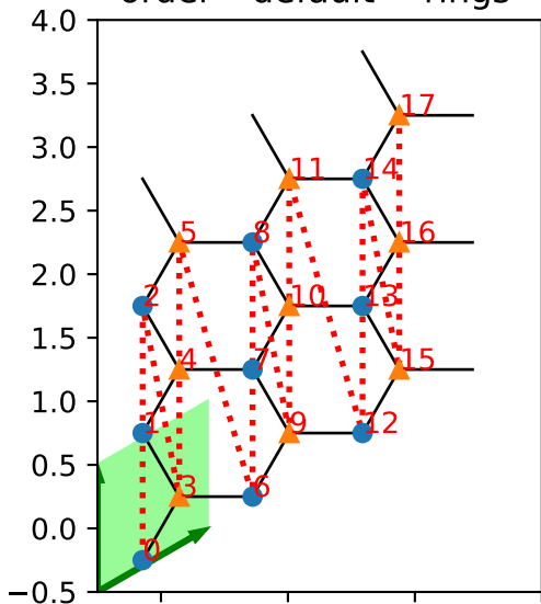
order='default'='rings'
