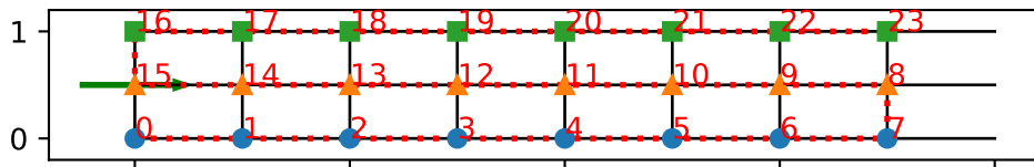
order='snakeFstyle'
