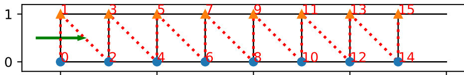
order='default'
