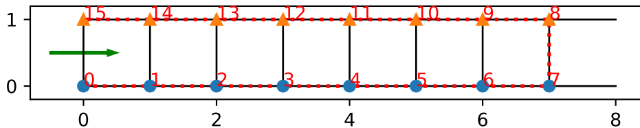
order='snakeFstyle'
