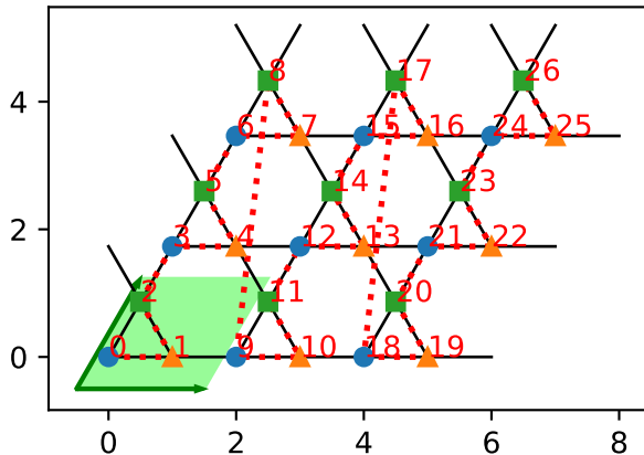
order='default'='Cstyle'
