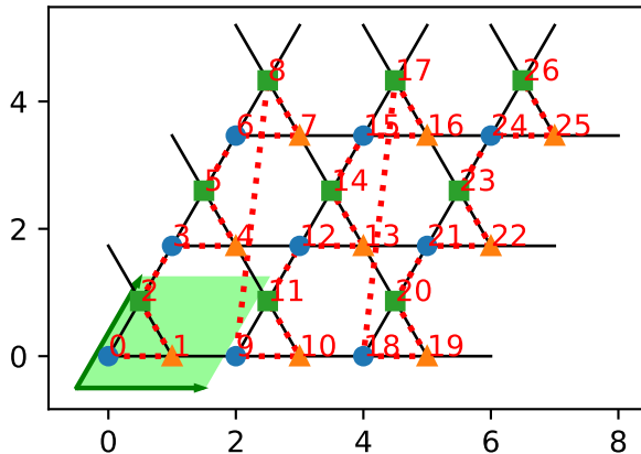
order='default'='Cstyle'
